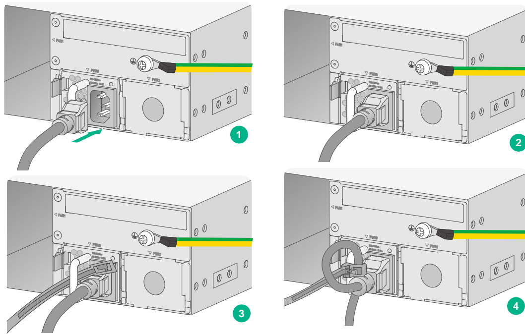
图2-16 连接交流电源线
