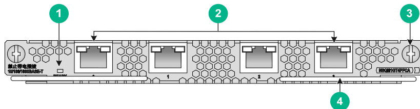
图A-5 NSQM1GT4PFCA 接口模块正视图
