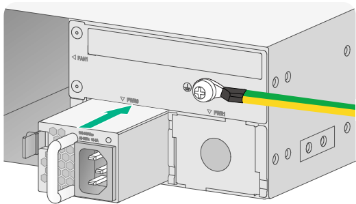
图2-6 安装电源模块（以交流电源模块为例）
