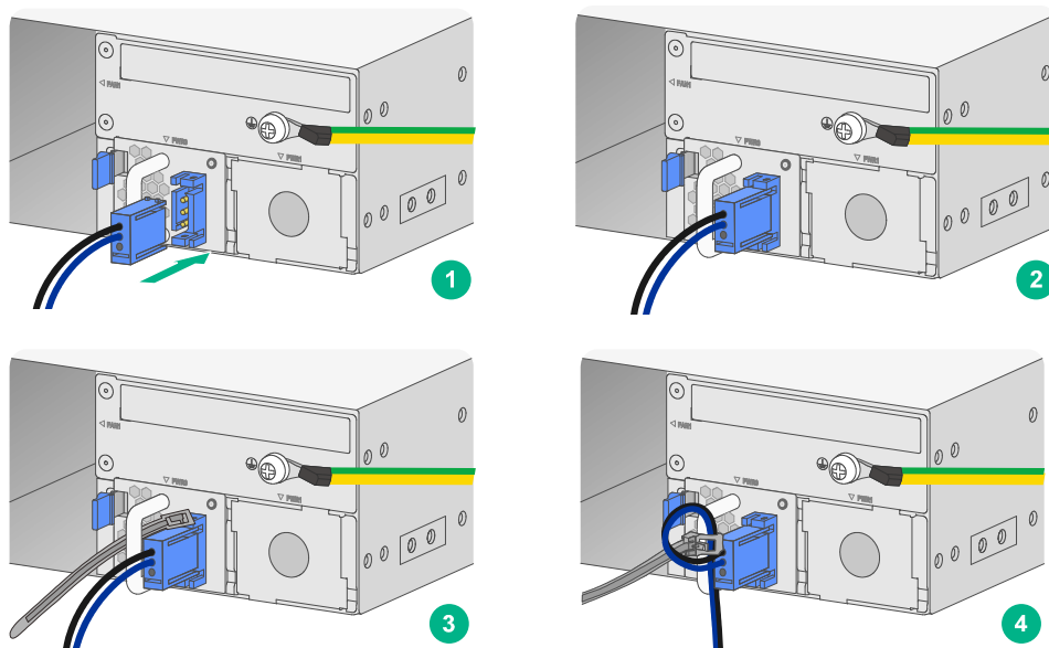
图2-17 连接直流电源线
