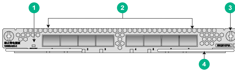
图A-6 NSQM1GP8A 接口模块正视图
