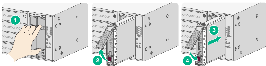
图2-10 安装硬盘
