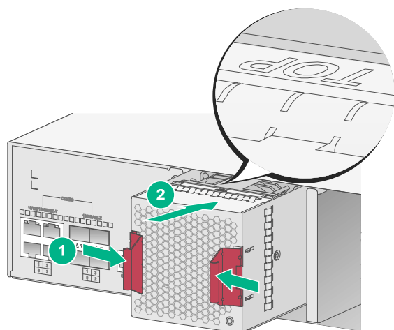
图2-8 风扇模块安装示意图
