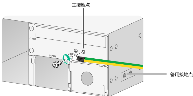
图2-5 连接接地线（以主接地点为例）
