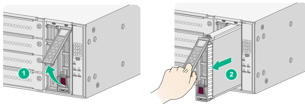
图2-11 拆卸硬盘
