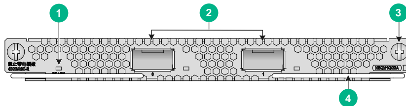
图A-7 NSQM1QG2A 接口模块正视图
