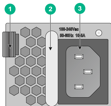
图A-9 交流电源模块正视图
