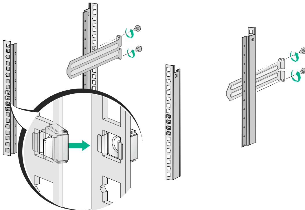
图2-2 安装浮动螺母及滑道
