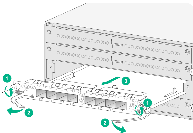
图4-4 拆卸 NSQM1GP8A 接口模块
