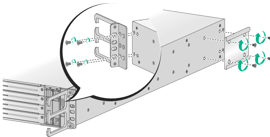
图2-3 安装前挂耳
