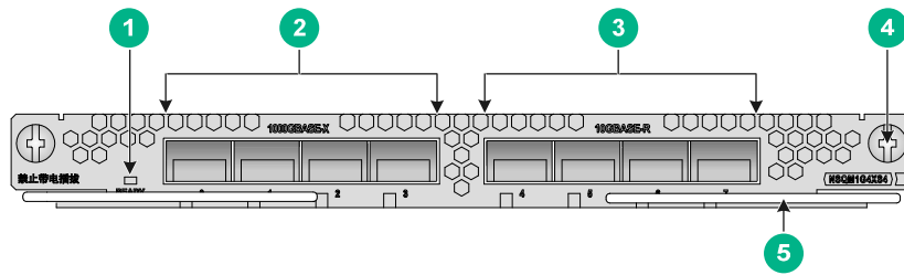
图A-3 NSQM1G4XS4 接口模块正视图
