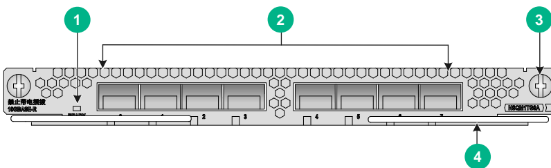
图A-8 NSQM1TG8A 接口模块正视图
