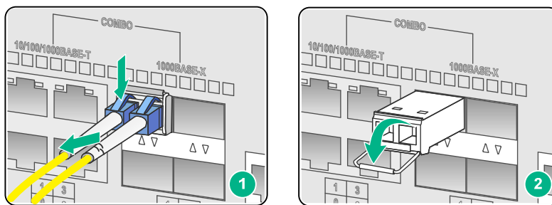
图4-6 拆卸光接口模块示意图
