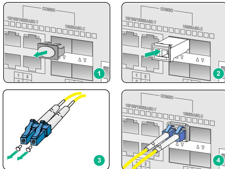
图2-15 安装及连接光模块
