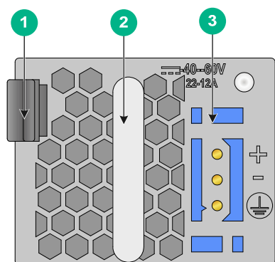
图A-10 直流电源模块正视图
