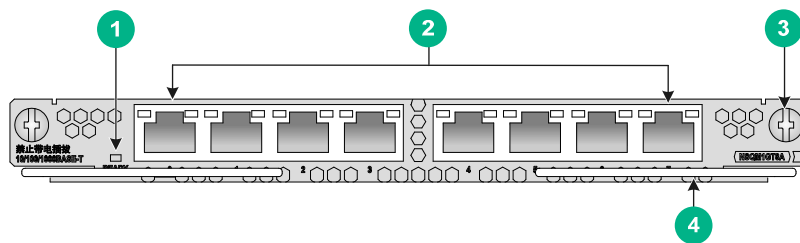
图A-4 NSQM1GT8A 接口模块正视图
