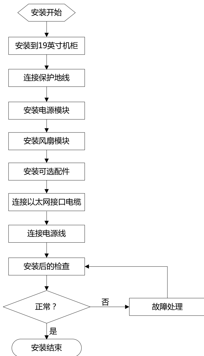
图2-1 设备安装流程示意图
