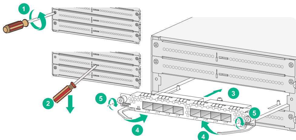
图2-9 安装 NSQM1GP8A 接口模块
