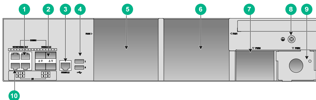
图A-2 设备后视图
