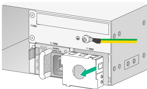
图2-7 拆卸电源槽位假面板
