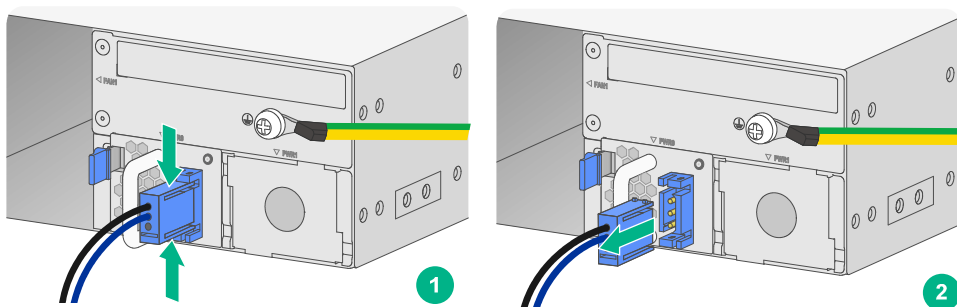
图4-2 拆卸电源线（以直流电源线为例）
